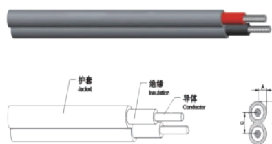
PV Cable
