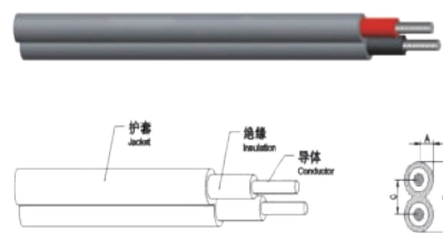
PV Cable
